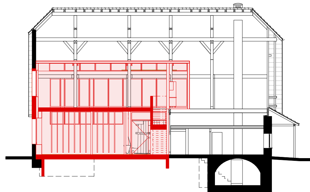
Längsschnitt
